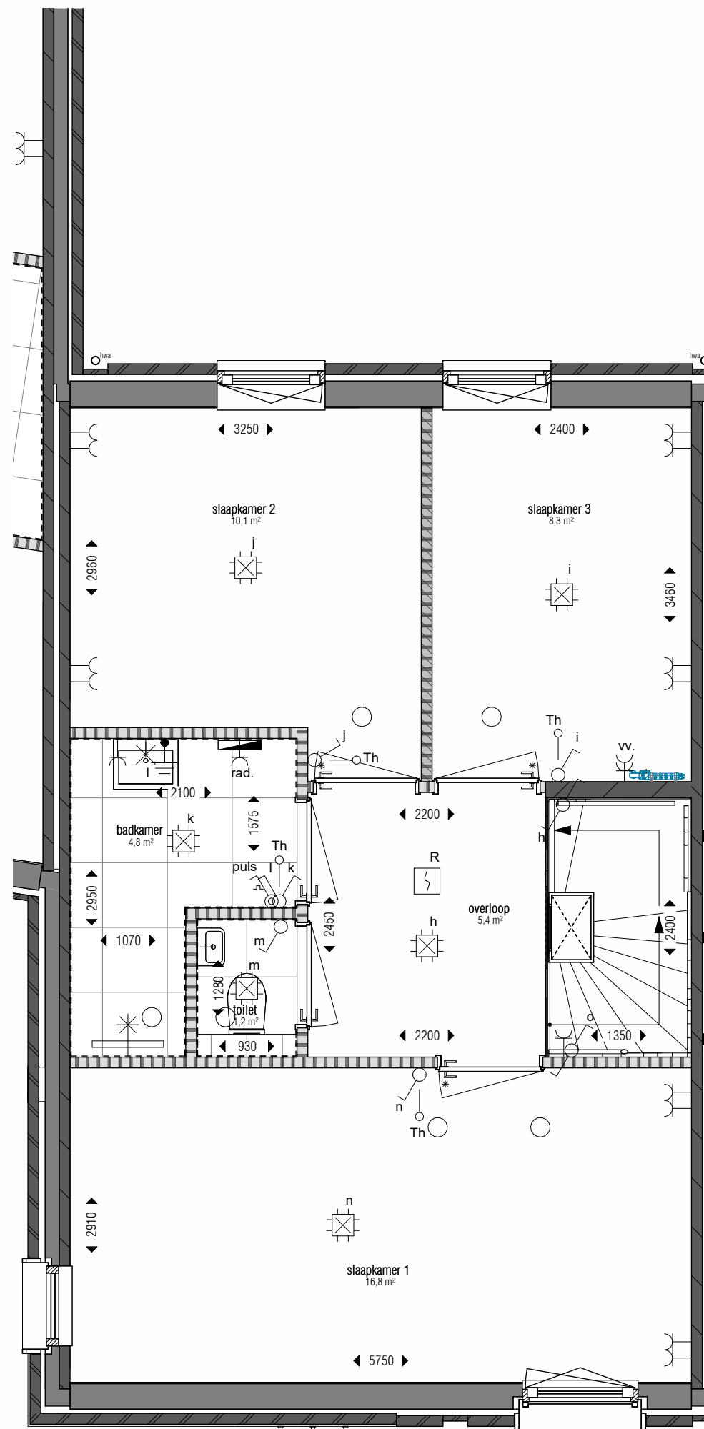
eerste verdieping 1 : 50
