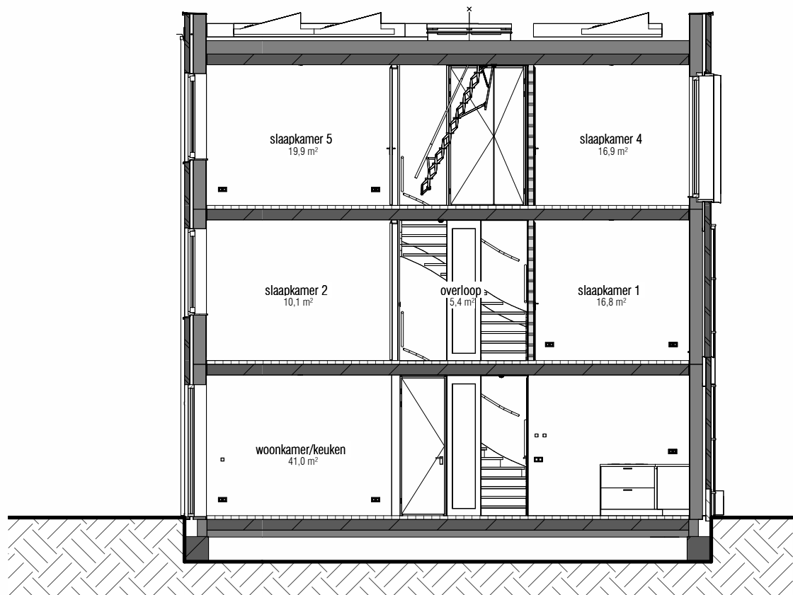
doorsnede 1 : 100
