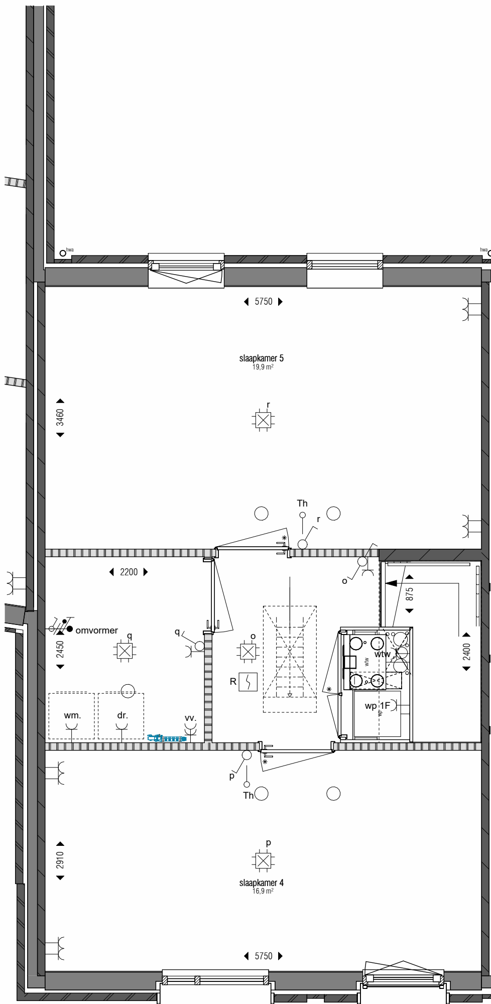
tweede verdieping 1 : 50
